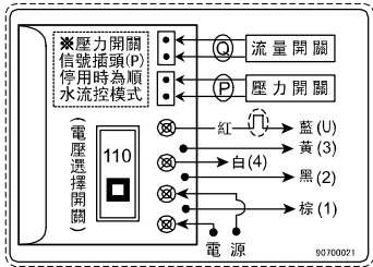
控制器結線圖
