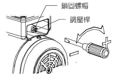
壓力開關調整
