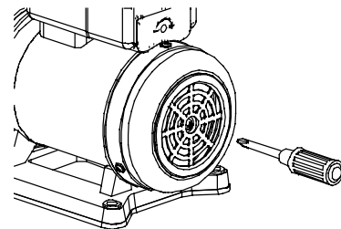
馬達主軸卡死檢查
